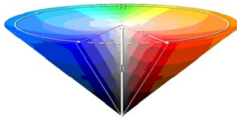
Abbildung 10: HSB Farbmodell
