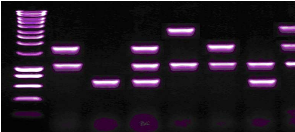
Abbildung 7: DNA-Fragmente im UV-Licht einer Elektrophorese [NYY05]
